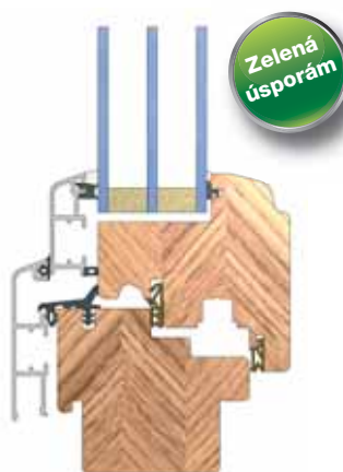
Řez okenním profilem EURO IV 78 (dřevohliník)
