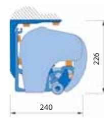
Montáž do stropu
