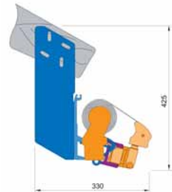
Montáž do krovu
