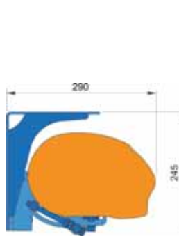
Montáž do stropu
