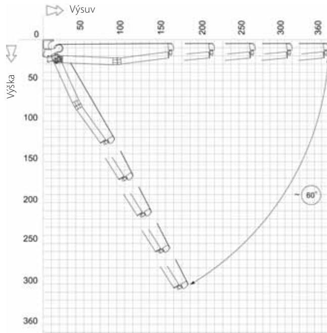
Rozsah regulace sklonu markíz
