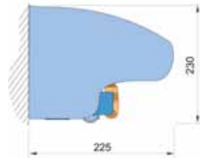
Montáž do zdi (verze se stříškou)
