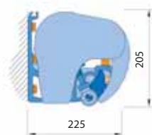
Montáž do stěny
