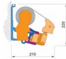
Montáž do stěny
