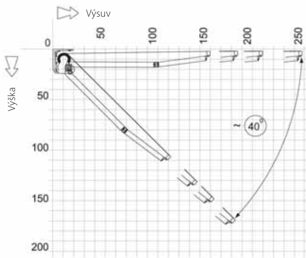
Rozsah regulace sklonu markýz
