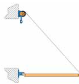
pohled z boku • markýza roztažená
