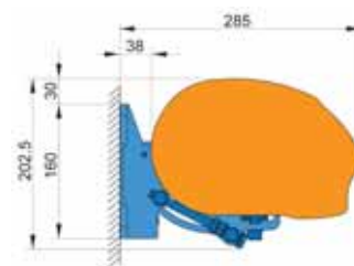
Montáž do stěny
