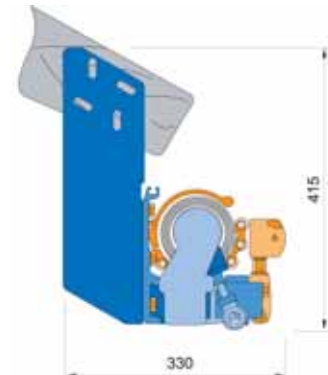
Montáž do krovu
