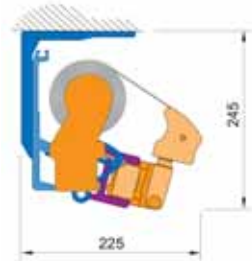
Montáž do stropu
